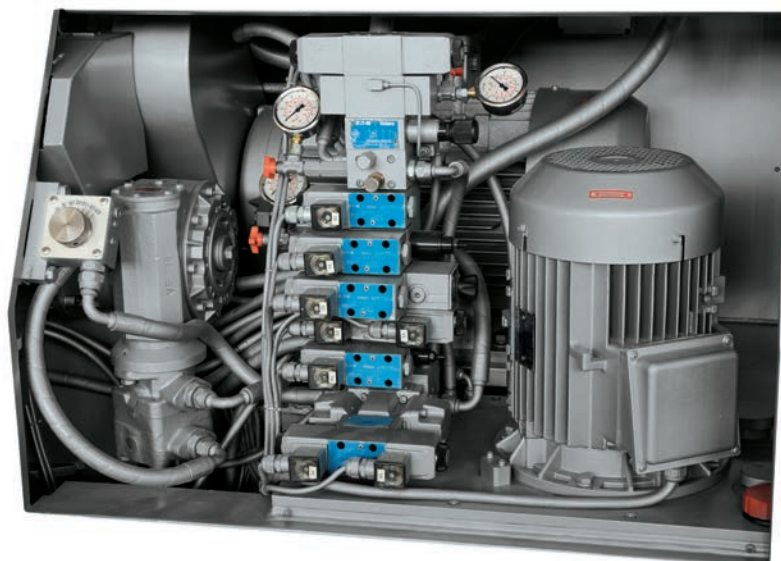
Particolare centralina idraulica Framming of hydraulic unit
